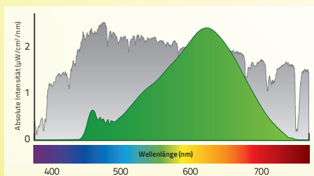
Das naturnahe Lichtspektrum der Pure-Z-NEO-LED
